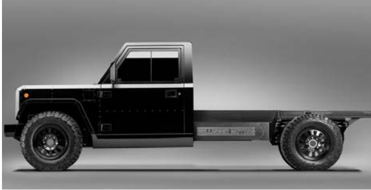
Afturhluti Bollinger B2 CC er þannig útbúinn að hægt verður að skipta út ýmsum gerðum búnaðar eins og yfirbyggingu, palli eða jafnvel krana.
