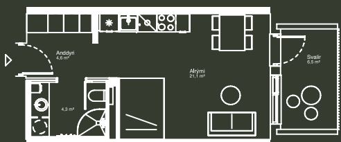
Stúdíóíbúð, 43 m 2
