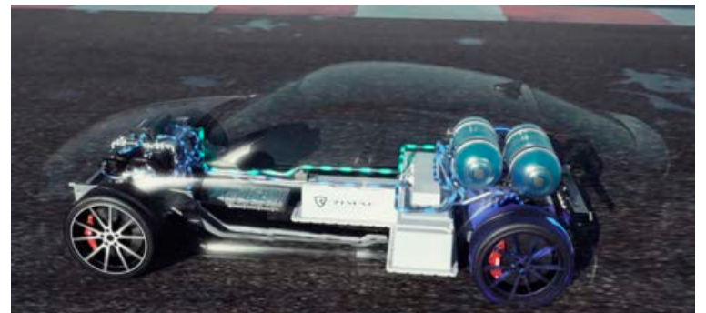
Myndin sýnir hvernig vetnisbúnaði og rafhlöðu er komið fyrir í bílnum.
